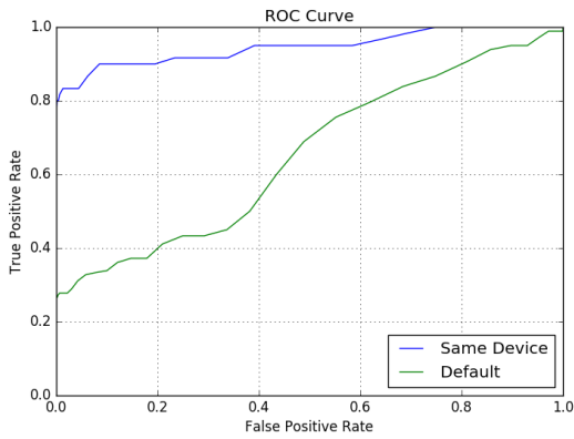
Fig. 3: Model 1 EQ ROC
